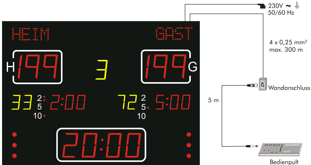
Abbildung mit Textdisplay (Option)
